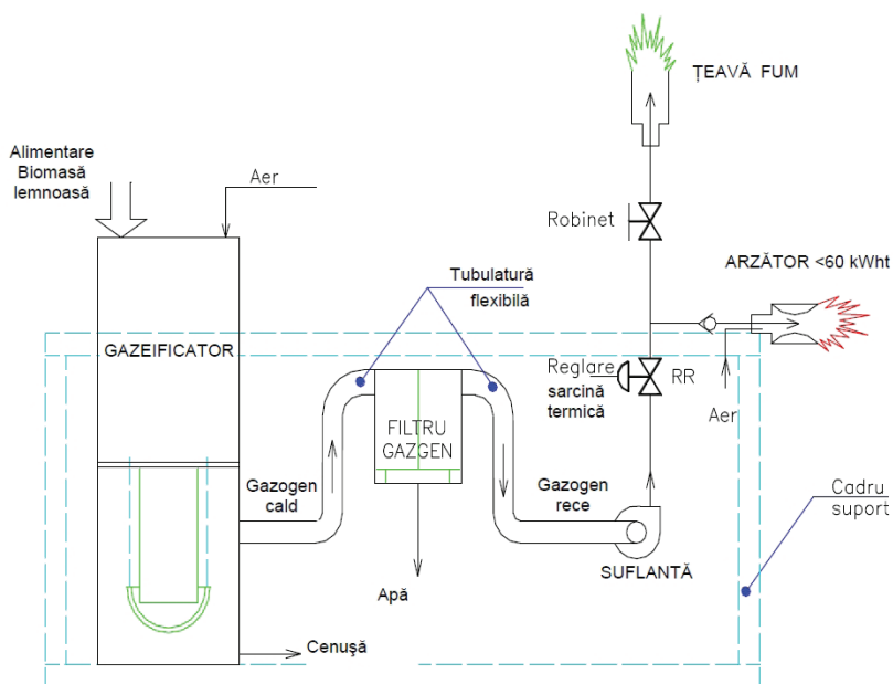
Figura 9. Schița instalației de gazeificare.
